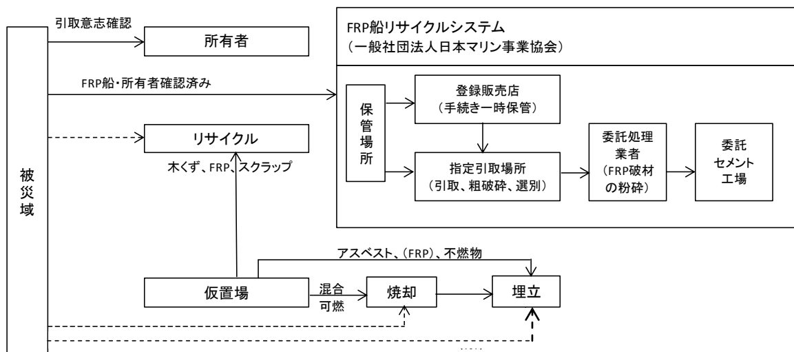
図 13 被災船舶の処理フロー
