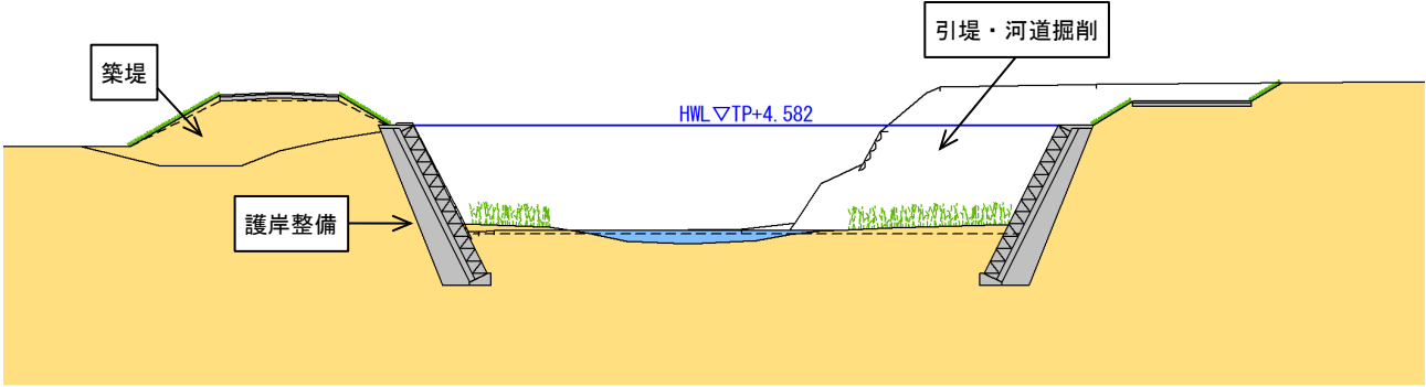
图 10 改修断面图
