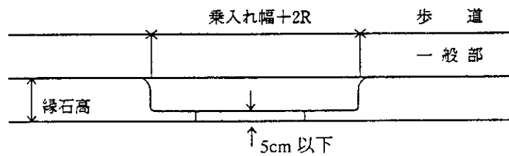
b—b' 正面図
