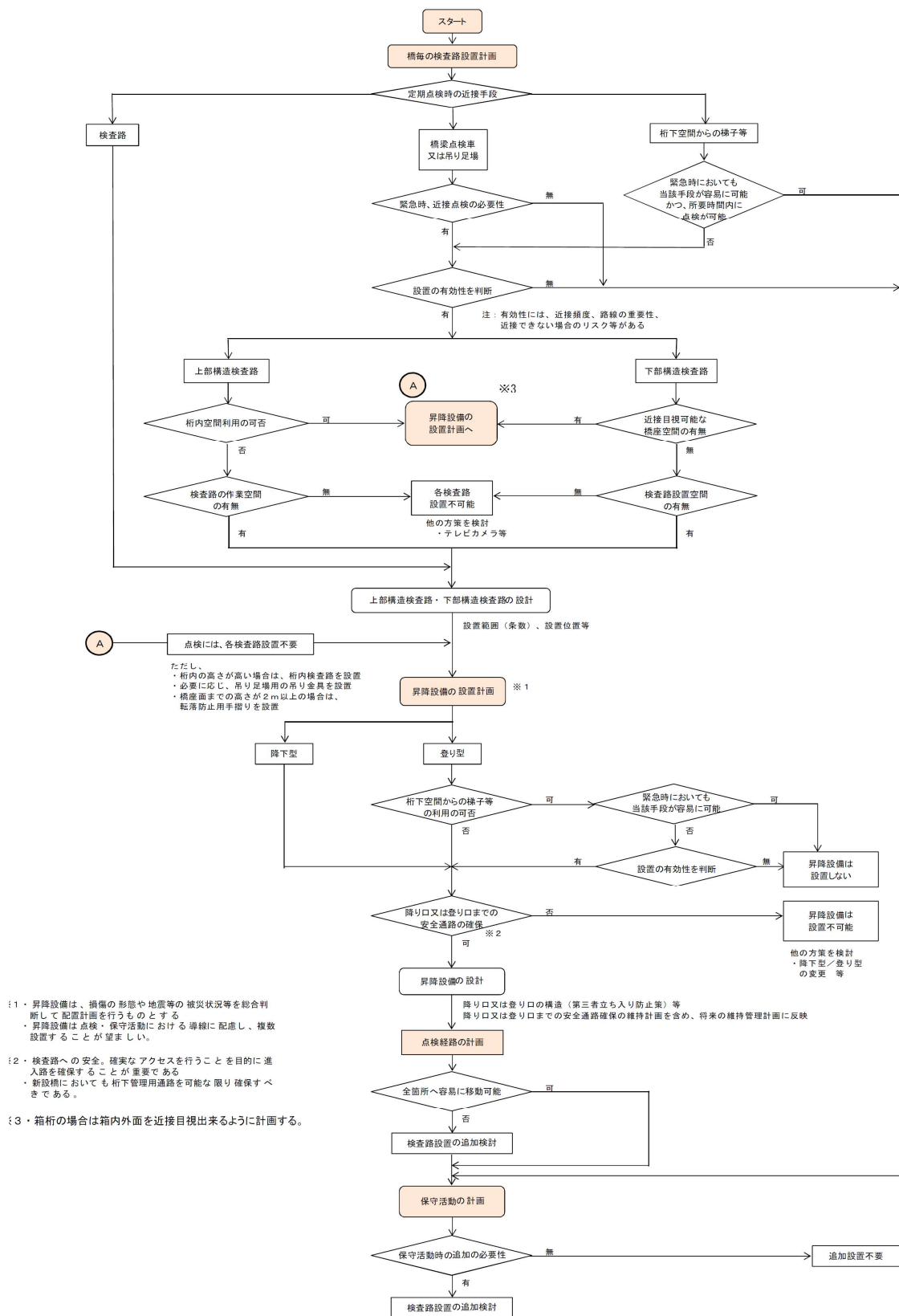
図-6-1 検査路の標準的設置判定フロー
