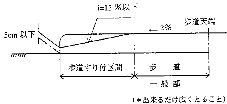
a—a' 断面図
