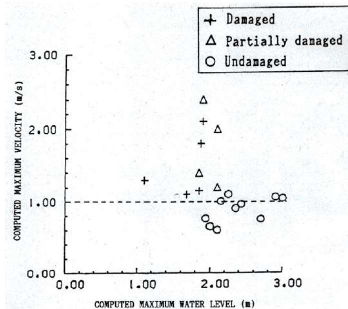
図 11.10-1 養殖筏の被害 (首藤 (1992) による経験則) エラー! ブックマークが定義されていません。
