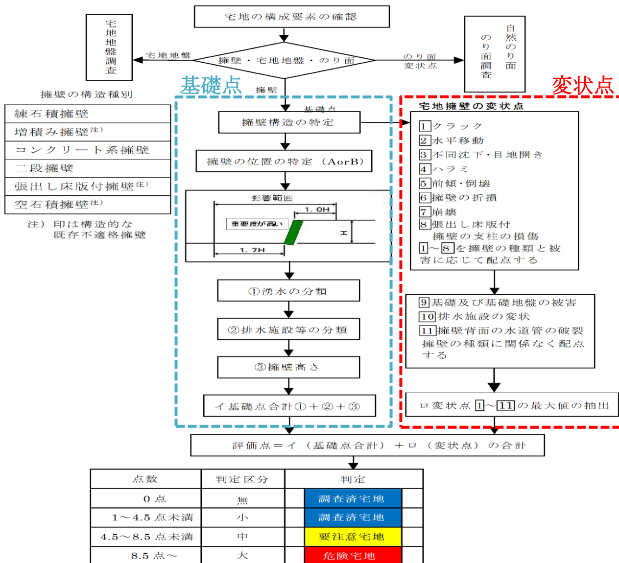
図3-2 擁壁の危険度判定フロー
