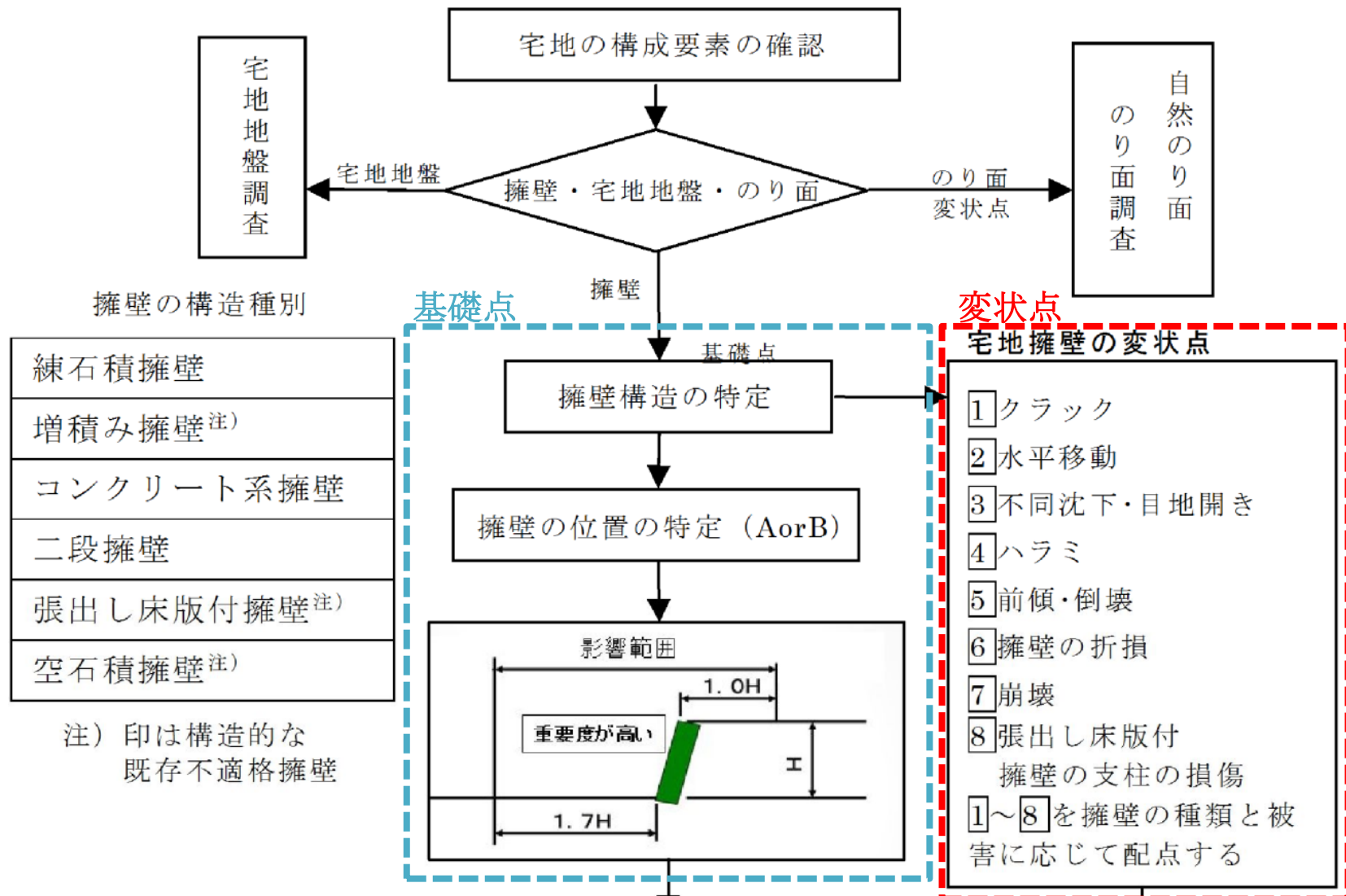
図3-2 擁壁の危険度判定フロー
