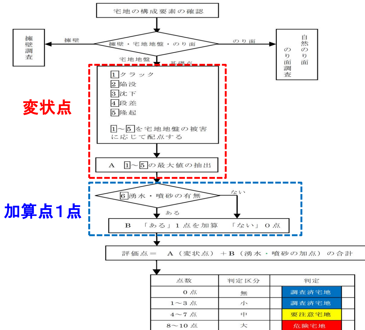
図3-6 宅地地盤の危険度判定のフロー
