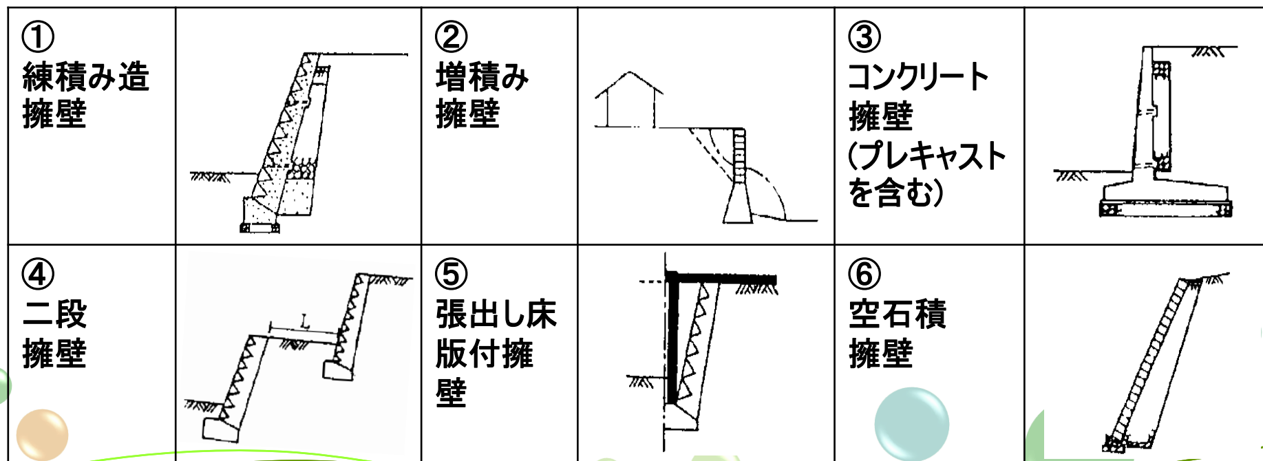
図3-2 擁壁の種類
