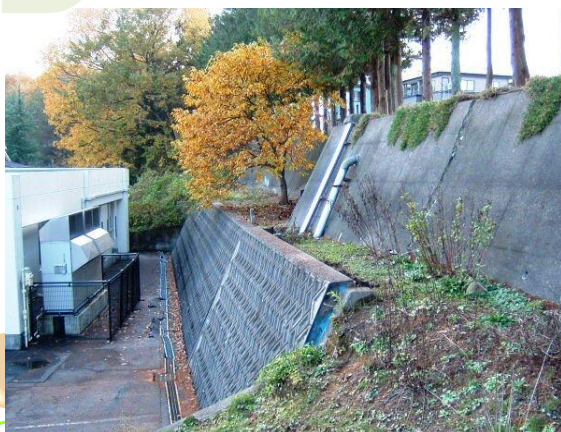
二段擁壁
